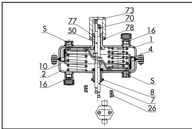
Fig. 14: Tipo 3271 com limitador de curso ajustável
