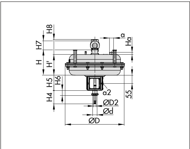
Fig. 27: Tipo 3277 com limitador de curso
