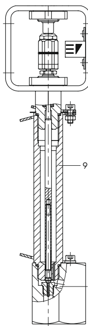
Bild 3: Stellventil Typ 3510, Eckventil mit Isolierteil
