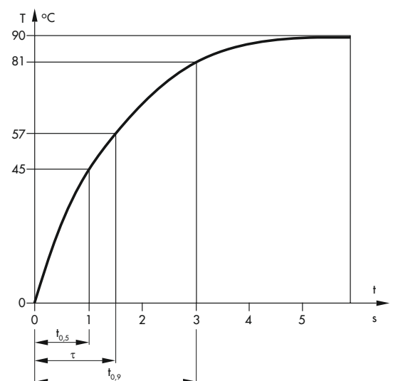
Bild 2: Übergangsfunktion
