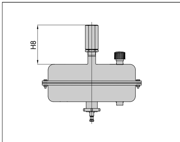
Fig. 4: 1400-60 cm 2 de área do atuador, com limitador de curso ajustável
