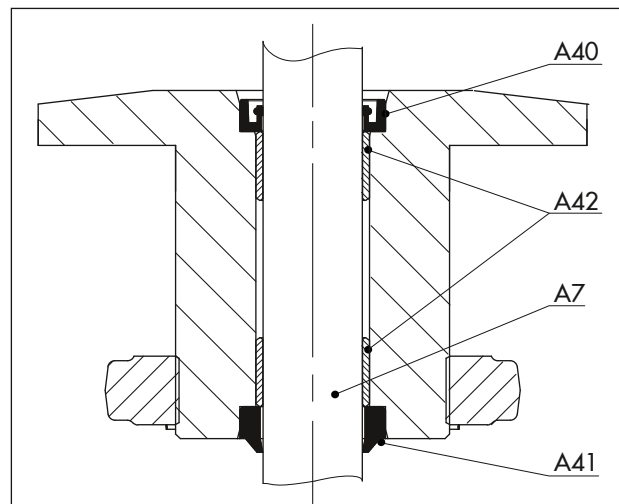
Fig. 17: Vedação da haste do atuador (Tipo 3271)
