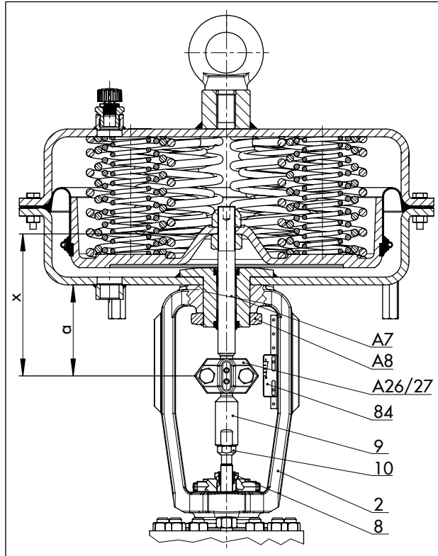
Fig. 8: Atuador pneumático Tipo 3271 montado numa válvula globo
