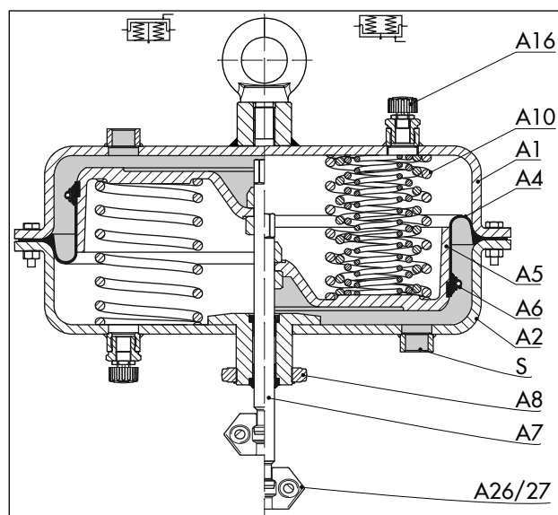
Fig. 12: Atuador pneumático Tipo 3271, desenho que apresenta um exemplo com área do atuador de 1400-60 cm 2
