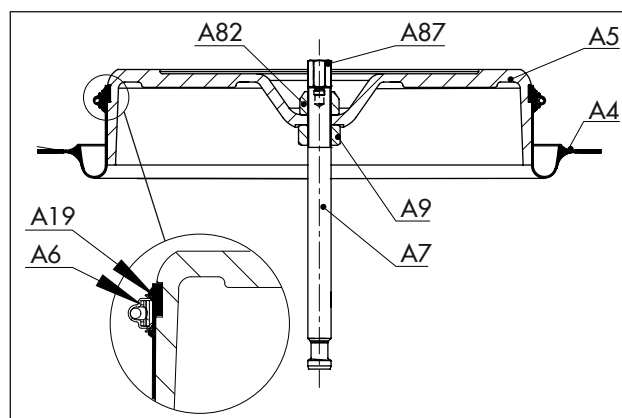
Fig. 15: Ordem das peças no sentido de ação «haste retrai» (1400-60 cm 2 )
