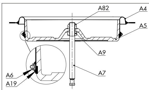
Fig. 13: Ordem das peças no sentido de ação «haste estende» (1400-60 cm 2 )
