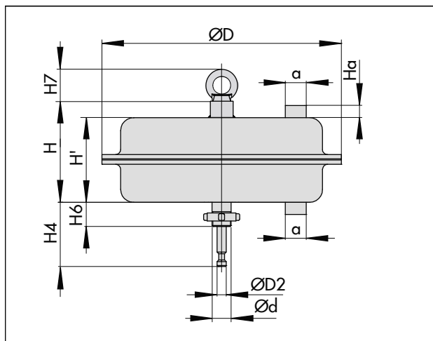
Fig. 3: Tipo 3271 com 1400-60 cm 2 de área do atuador
