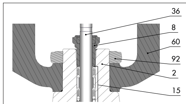
Fig. 22: Empanque com casquilho roscado (fixação centralizada) (exemplo apresentado)
