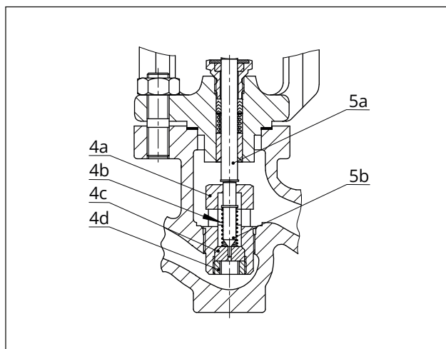
Fig. 6: Obturador microcaudal
