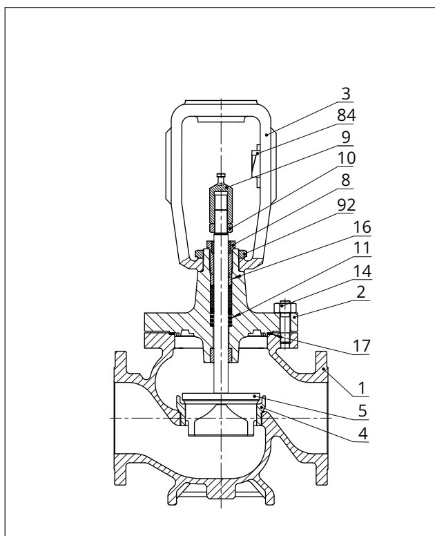
Fig. 5: Válvula Tipo 3241, corpo DN 200 a 300/NPS 8 a 12
