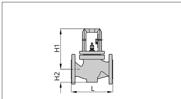
Fig. 13: Tipo 3241 · Tamanhos nominais até DN 150/NPS 6/ DN 150A
