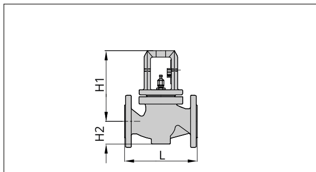
Fig. 7: Tipo 3241 · Tamanhos nominais até DN 150/NPS 6/ DN 150A
