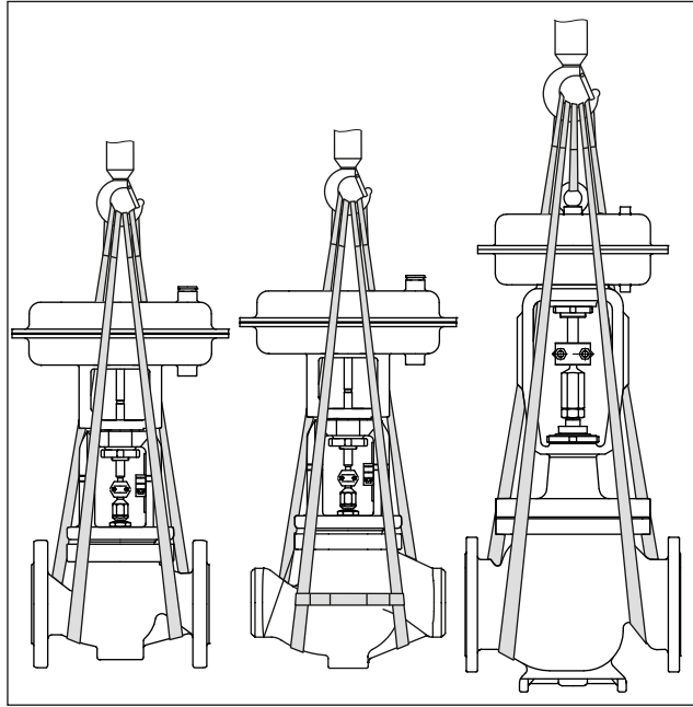
Fig. 14: Pontos de elevação na válvula de controlo: até DN 150/NPS 6 com flanges (esquerda) e com extremidades para soldar (meio) · DN 150/NPS 6 e superior com olhal de elevação adicional no atuador (direita)
