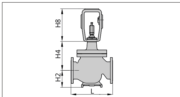
Fig. 8: Tipo 3241 · Tamanhos nominais até DN 200/NPS 8 e superior
