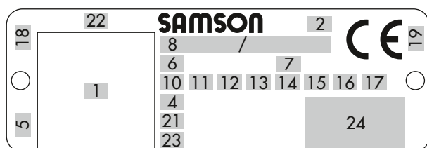
Fig. 2: Inscrições na placa de identificação da válvula
