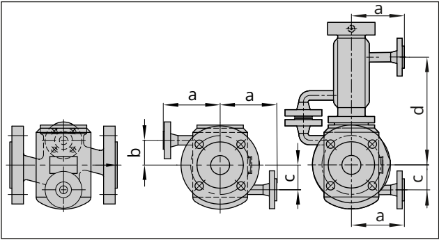
Fig. 12: Tipo 3241 com camisa de aquecimento, tamanho nominal DN 150/NPS 6 e superior · Com secção isolante ou fole de vedação (direita)
