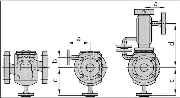
Fig. 11: Tipo 3241 com camisa de aquecimento até ao tamanho nominal DN 100/NPS 4 · Com secção isolante ou fole de vedação (direita)
