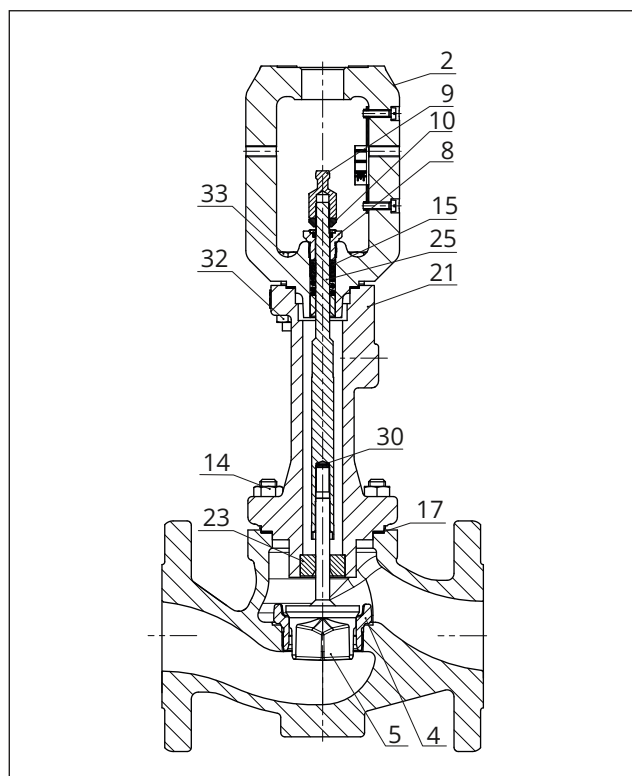
Fig. 25: Tipo 3241, versão com secção isolante
