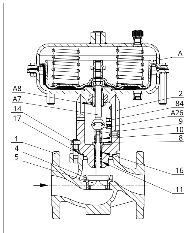
Fig. 24: Válvula de controlo Tipo 3241-1 com atuador pneumático Tipo 3271, corpo até DN 150/NPS 6
